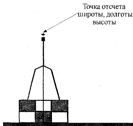
Рис. 7. Точки геодезической привязки VOR/DME.
